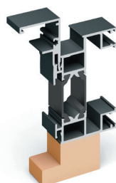
Standard : Tapée extérieure rapportée pour isolation de 90 à 200 mm
