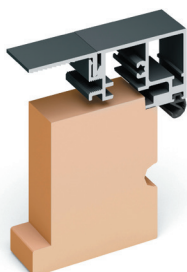
Oscillo coulissant : Dormant avec aile intégrée de 10mm
